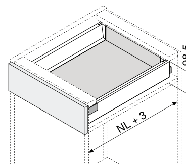
Menovitá dĺžka
