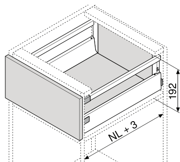
NL Menovitá dĺžka
