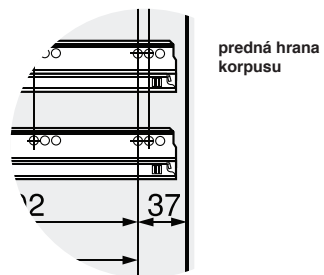
Montážne rozmery čela
