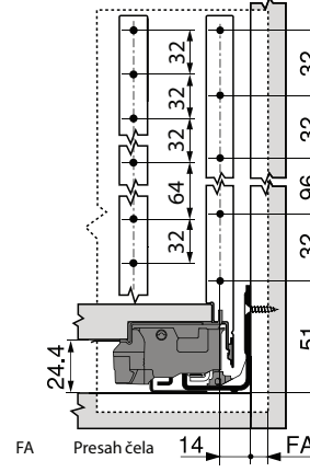
Montážne rozmery čela
