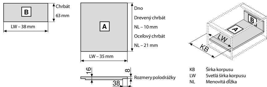
Prírez - 16 mm drevotrieskové dosky
