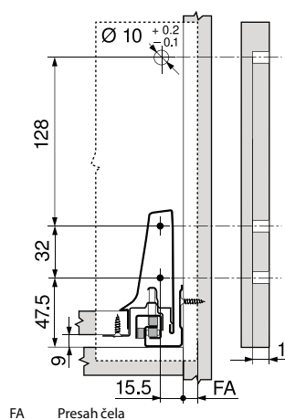
FA Presah čela
