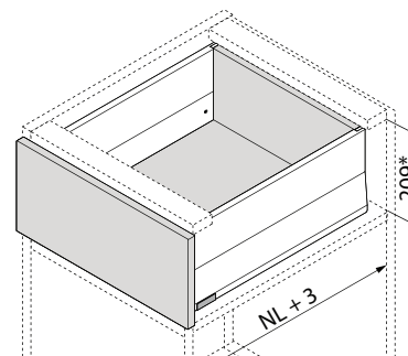
Potreba miesta v korpusu
