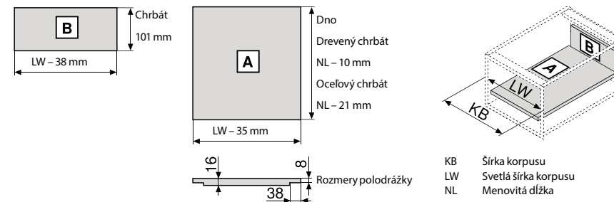
Prírez - 16 mm drevotrieskové dosky
