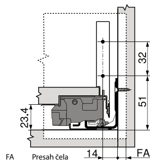
Montážne rozmery čela
