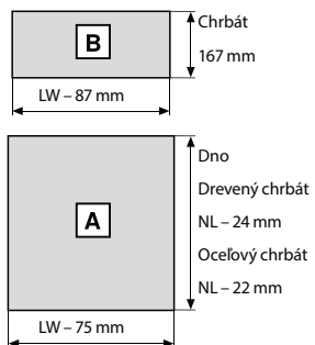
Prírez - 16 mm drevotrieskové dosky
