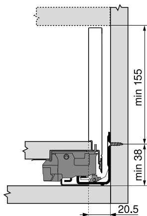
Prírez - 16 mm drevotriestkové dosky
