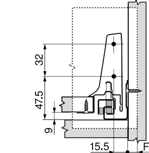
FA Presah čela
