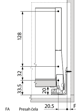
Montážne rozmery čela
