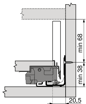
Prírez - 16 mm drevotrieskové dosky
