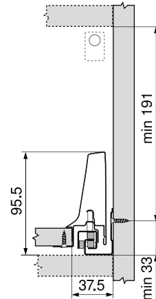
Prírez - 16 mm drevotrieskové dosky
