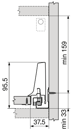
Potreba miesta v korpusu
