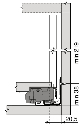
Prírez - 16 mm drevotriestkové dosky
