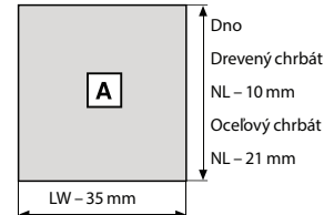
Prírez - 16 mm drevotriestkové dosky
