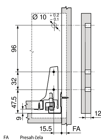
FA Presah čela
