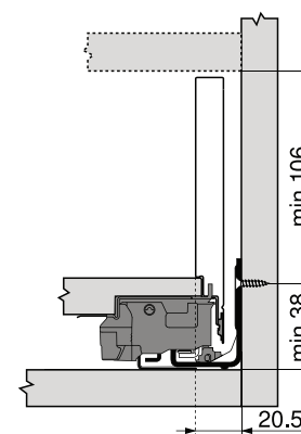
Prírez - 16 mm drevotrieskové dosky
