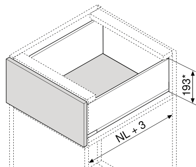
Potreba miesta v korpusu
