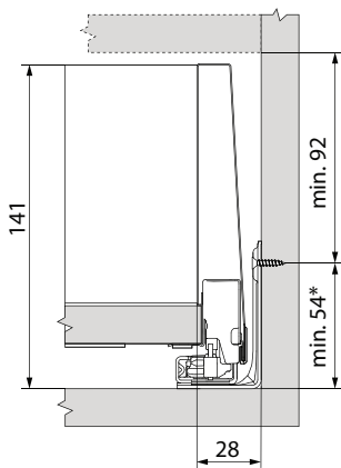
Prírez - 16 mm drevotrieskové dosky
