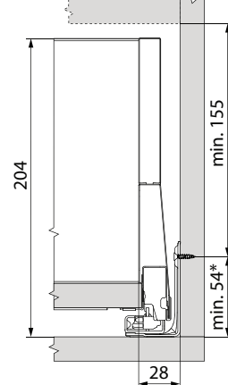
Prírez - 16 mm drevotrieskové dosky
