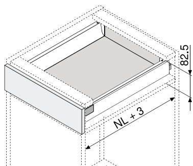
NL Menovitá dĺžka
