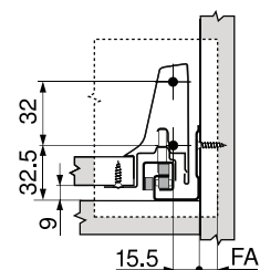
FA Presah čela
