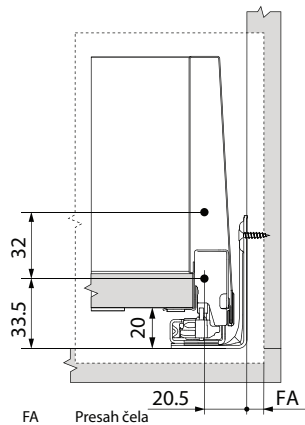
Montážne rozmery čela
