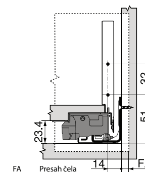
Montážne rozmery čela
